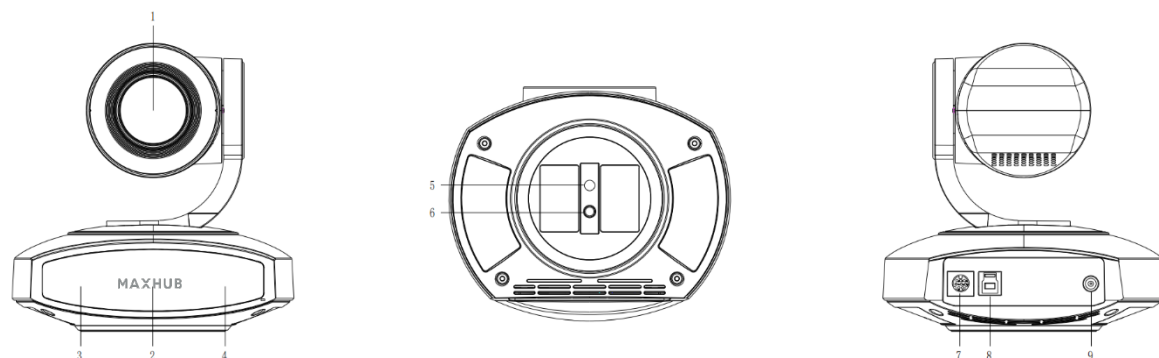
图 1-1 产品接口
