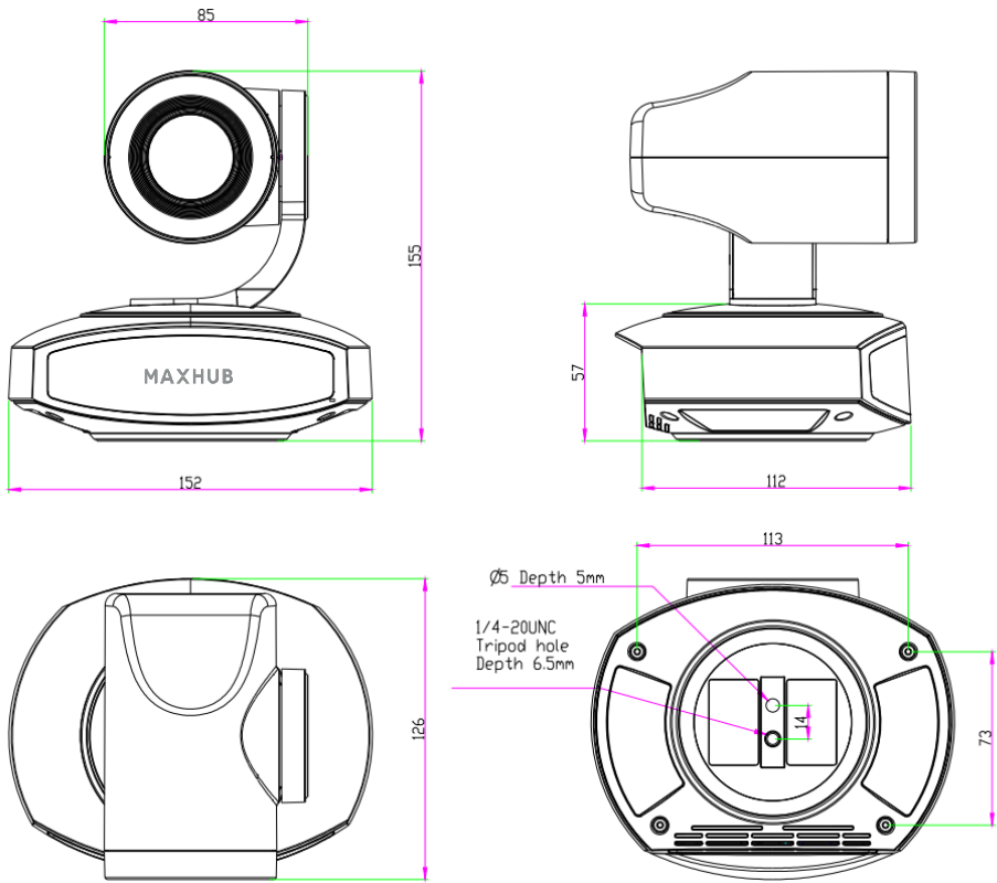
图 2-1 外型尺寸
