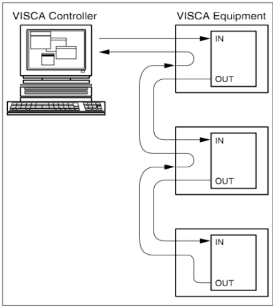
图 2-4 VISCA 组网方式示意图
