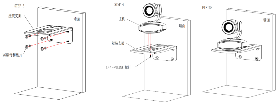
图 1-2 支架正装步骤
