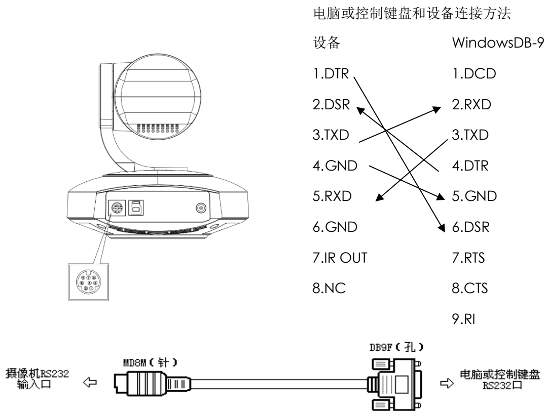
图 2-3 RS-232 接口示意图
