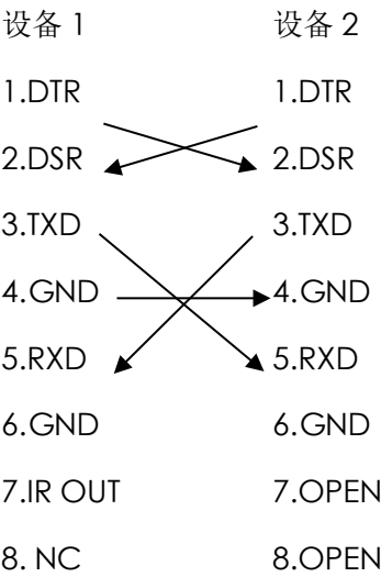
设备级联方式连接方法
