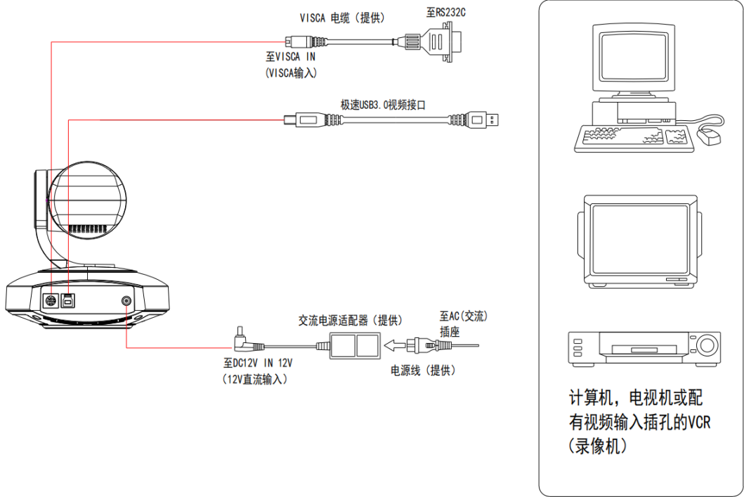
图 2-2 外部接口示意图
